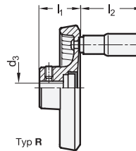
Příklad montáže
